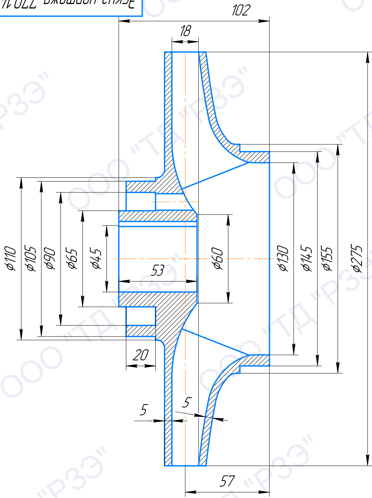
Эскиз чертежа 770.148
